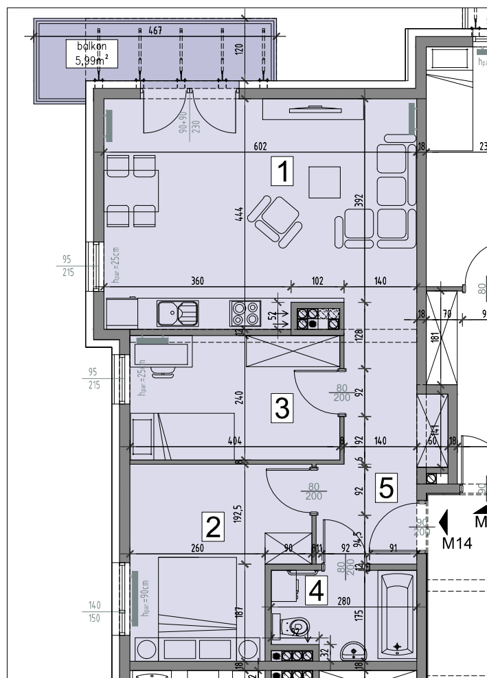
Uwaga: Wymiary na rysunku podano w stanie surowym
